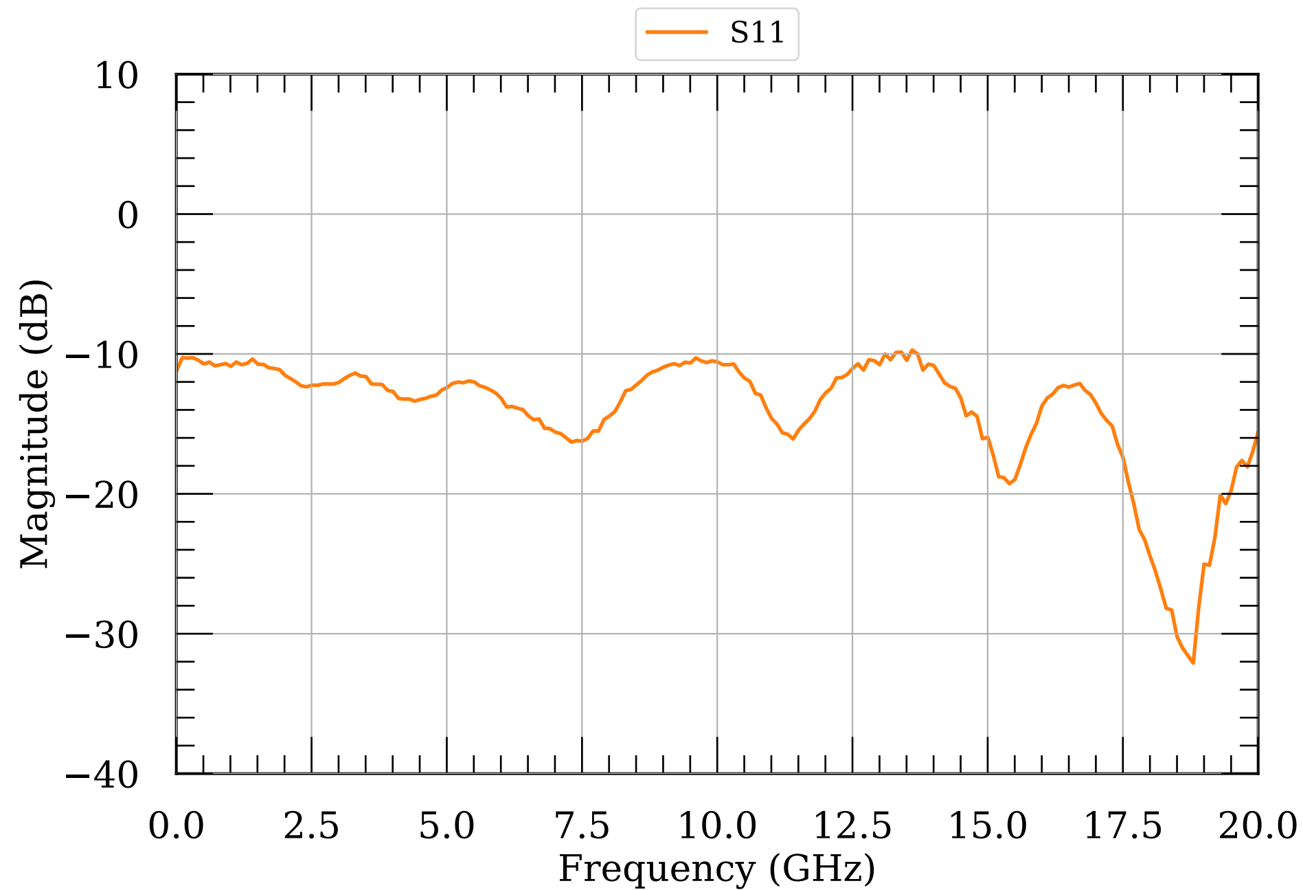
LNA S-params module081
